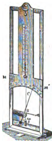
Č. 1870. Hygrometr vlasový.
